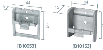
코너클립 | B10053/B10153
