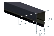
마감후레싱 | B254xxx
